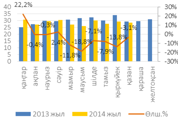
Мырыш концентратындағы, мың тонна
