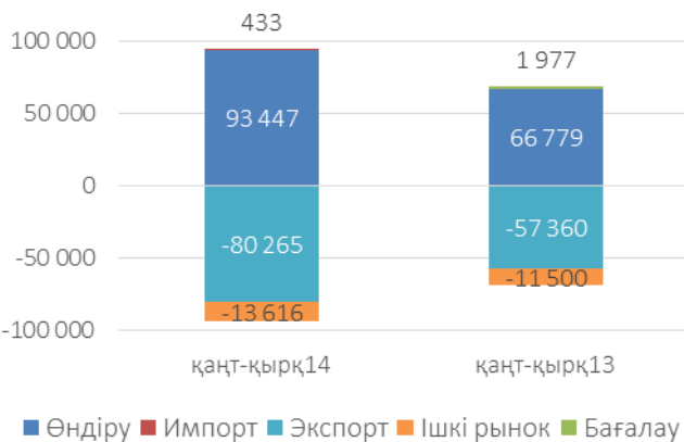
Ресурстар балансы және пайдалану: ҚОРҒАСЫН, тонна
