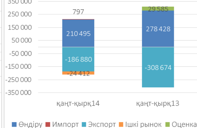
Ресурстар балансы және пайдалану: МЫС, тонна
