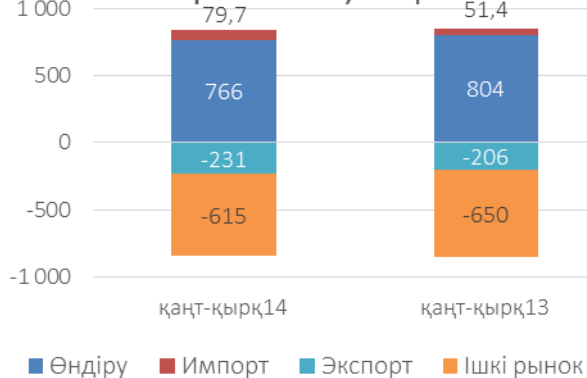
Ресурстар балансы және пайдалану: МЫРЫШ РУДАСЫ ЖӘНЕ КОНЦЕНТРАТТАР, мың тонна
