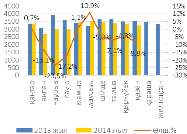
Мыс рудасын өндіру, мың тонна
